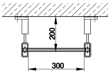
Ausführung schwer LL.AS
