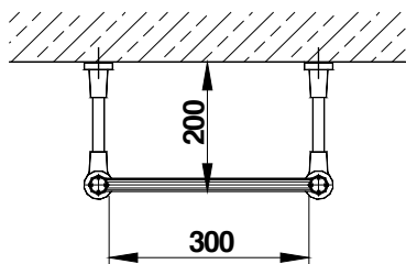
Ausführung leicht LL.AL
